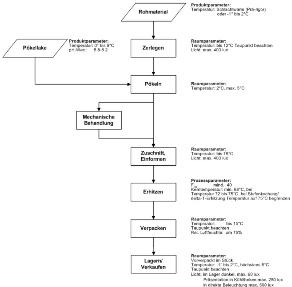
Abbildung 10: Fließdiagramm für die Kochschinkenherstellung
