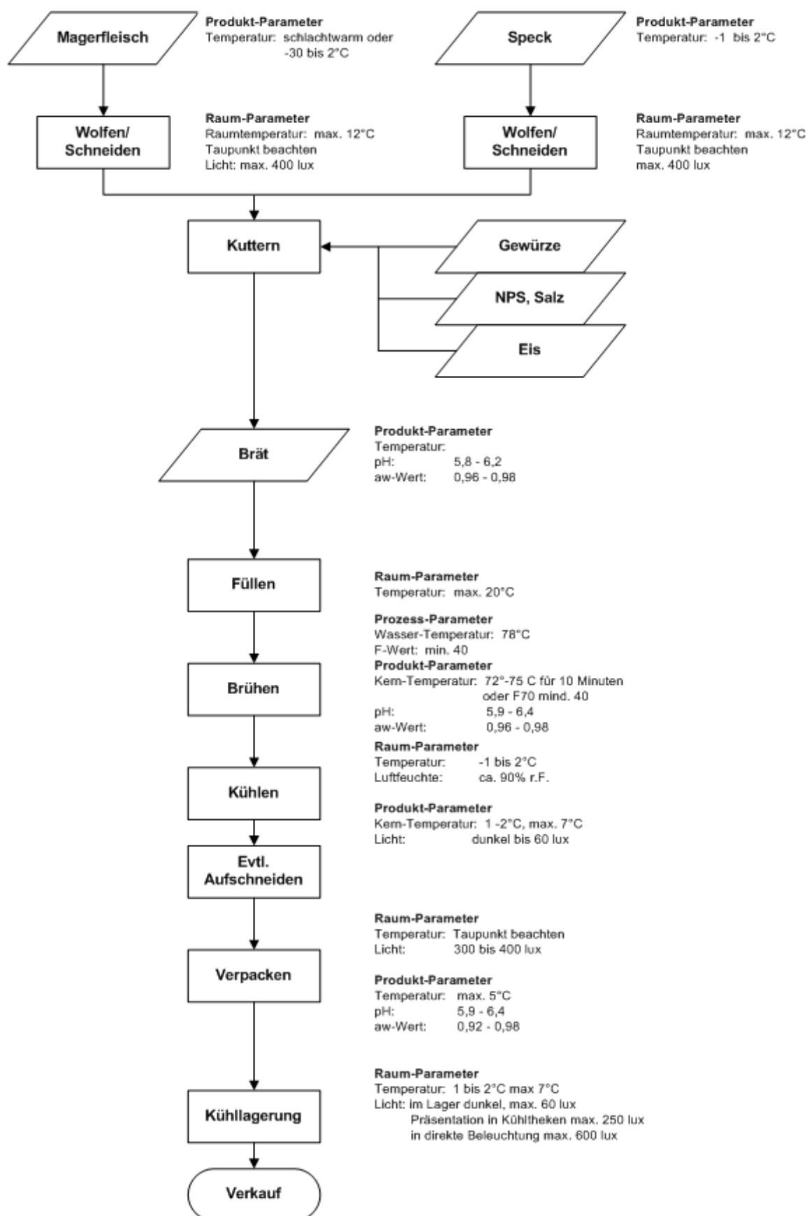
Abbildung 5: Herstellungsschema für Brühwürste
